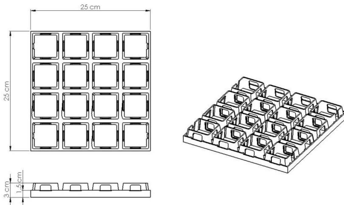
Figura 1: Dimensões.
